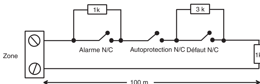
Figure 2-10. Option 09 - Câblage de surveillance des défauts boucle équilibrée 1k
