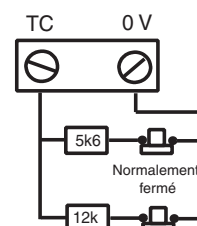
Raccordement du contact d'autoprotection
