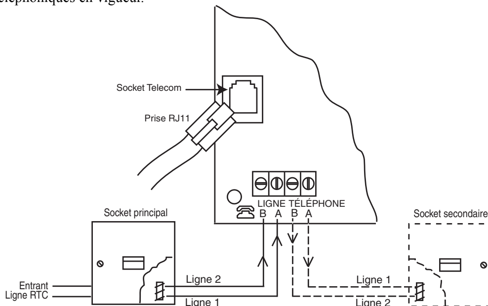
Figure 2-5. Raccordement de la centrale d'alarme Galaxy Dimension au réseau téléphonique
