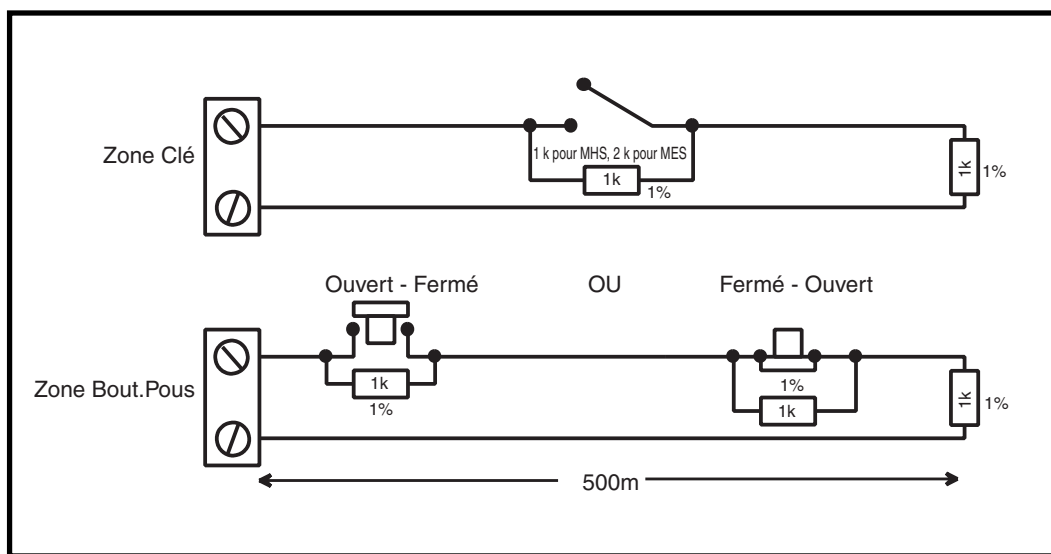
Figure 2-14. Câblage du terminateur à la zone Clé
