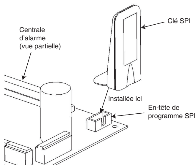
Figure 2-19. Connexion de la SPI KEY sur l'embase de programme
