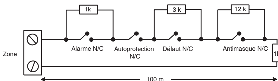
Figure 2-11. Option 09 - Câblage de surveillance de défaut 1 k/antimasque boucle équilibrée
