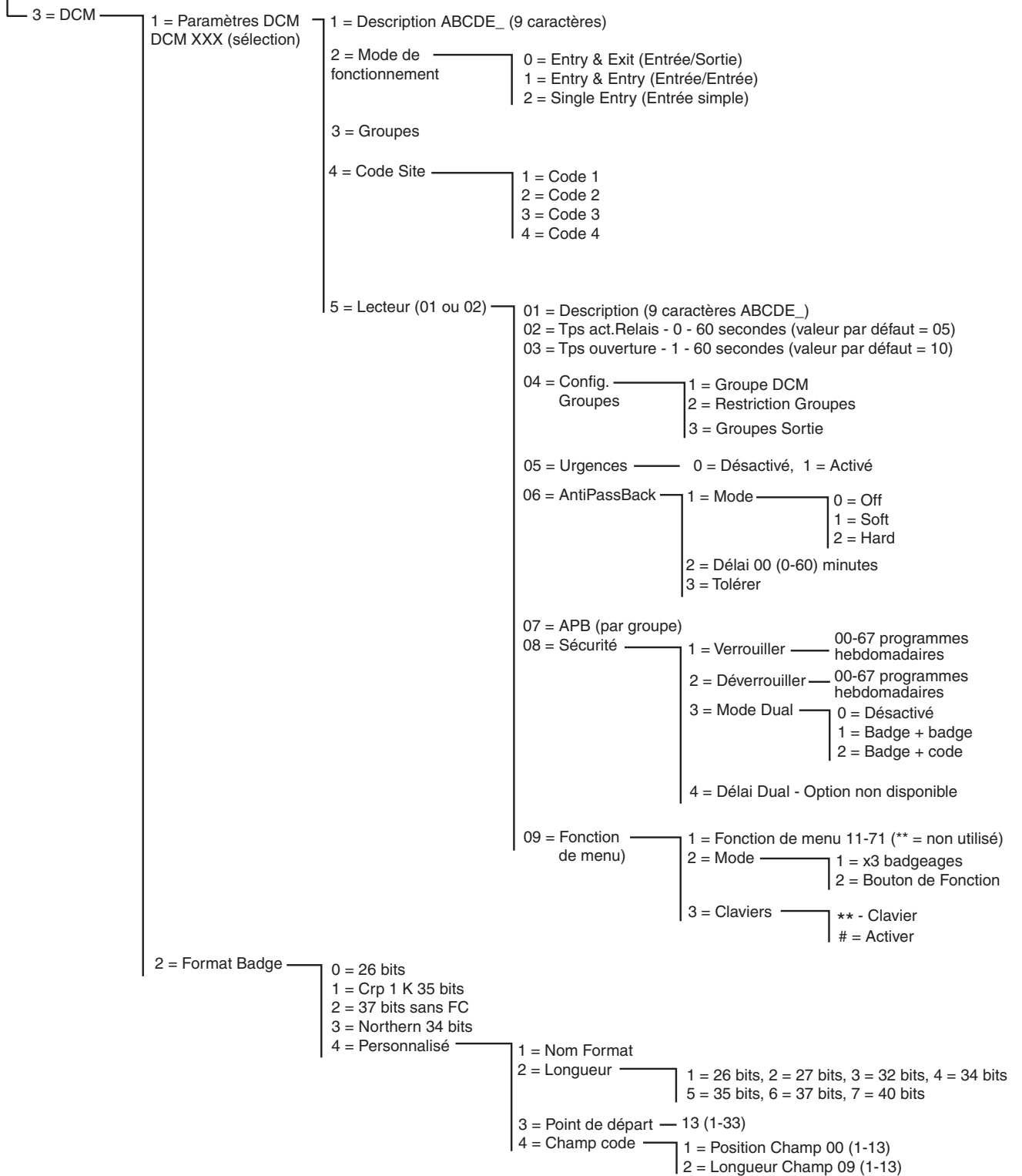
Figure 6-15. Structure de programmation du contrôle d'accès (page 2)
