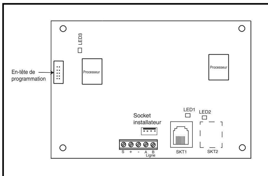
Figure 3-5. Présentation de la carte électronique Ethernet
