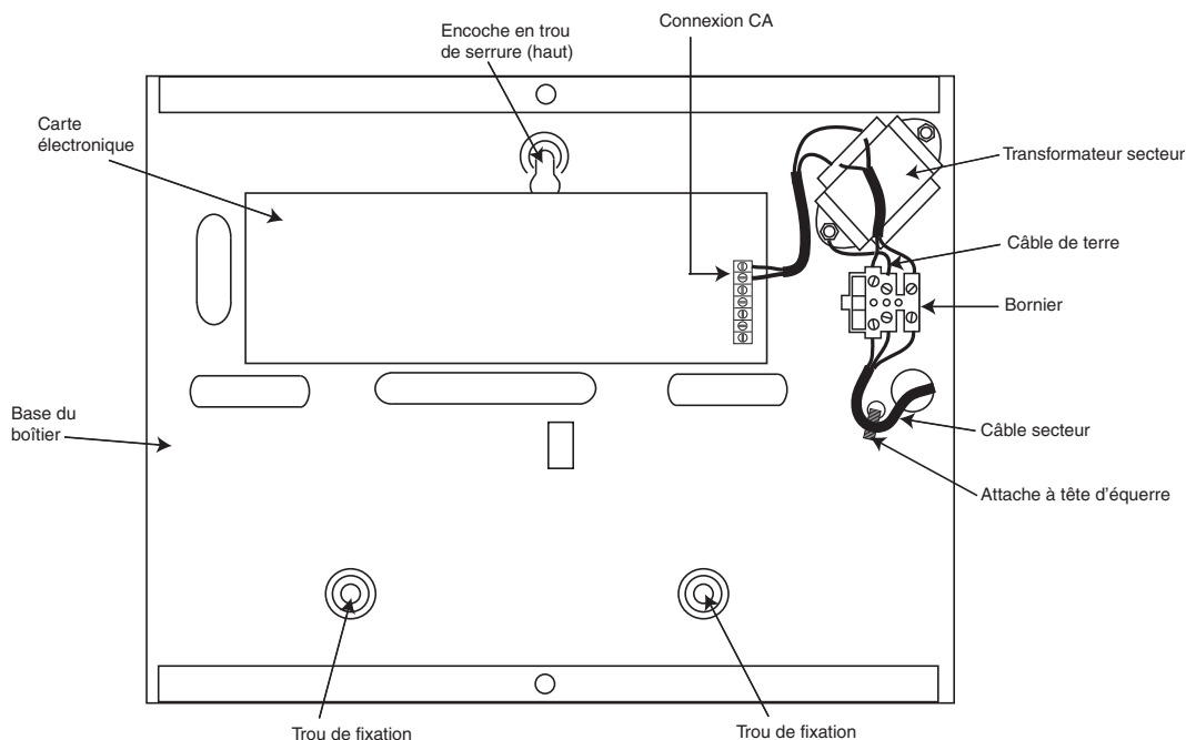
Figure 2-4. Fixation du câble d'alimentation sur la base du boîtier
