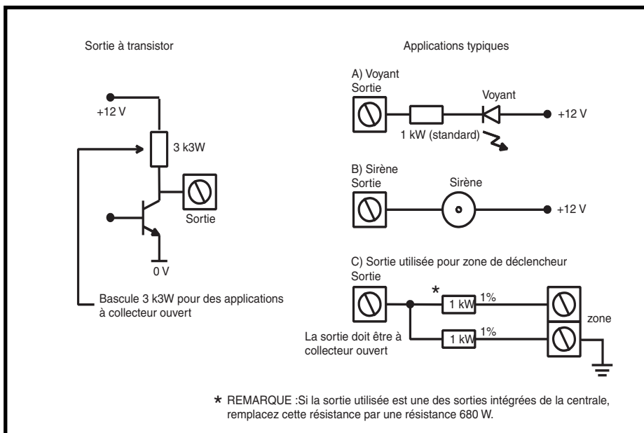
Figure 2-15. Configuration de sortie et applications standard
