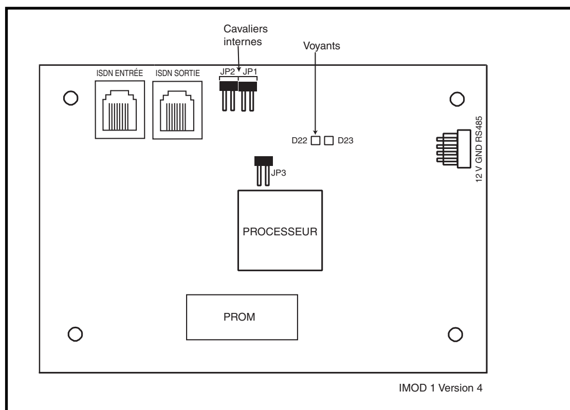
Figure 3-4. Présentation de la carte électronique ISDN
