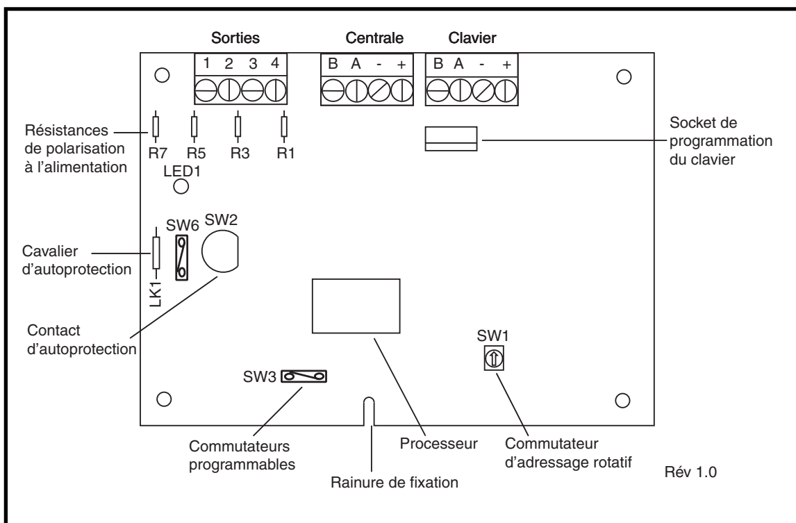
Figure 3-1. Présentation de la carte électronique RIO RF
