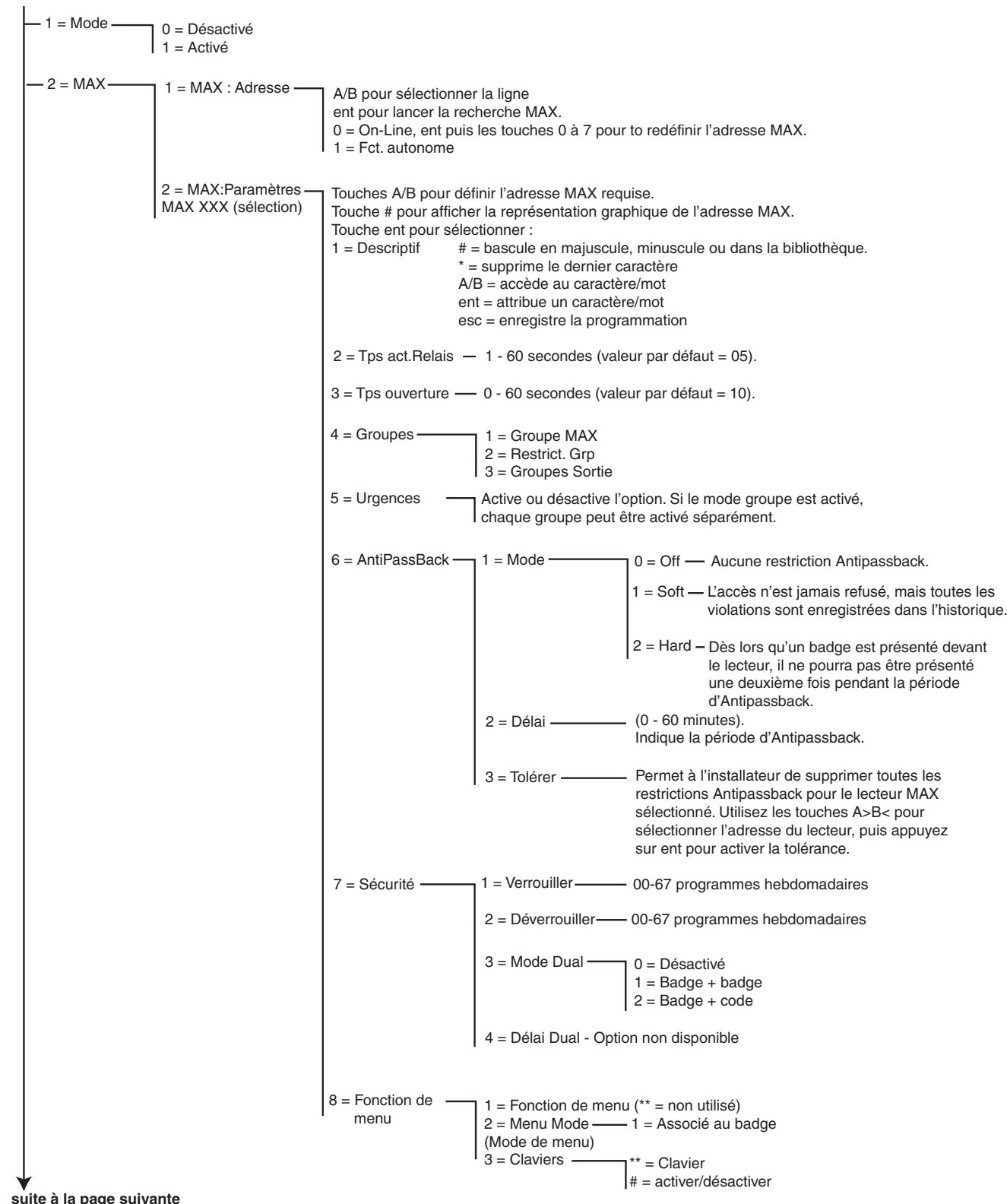
Figure 6-14. Structure de programmation du contrôle d'accès (page 1)
