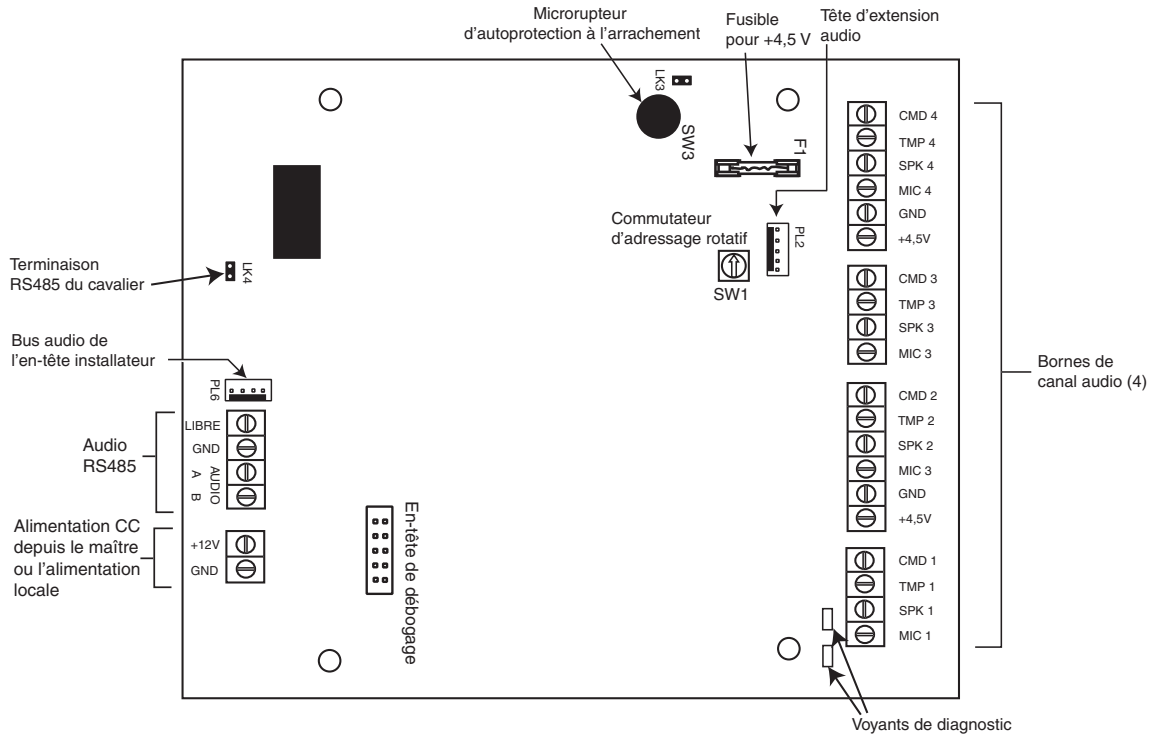
Figure 3-8. Carte électronique du module MUX
