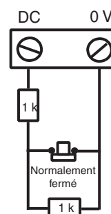
Raccordement du contact de porte
