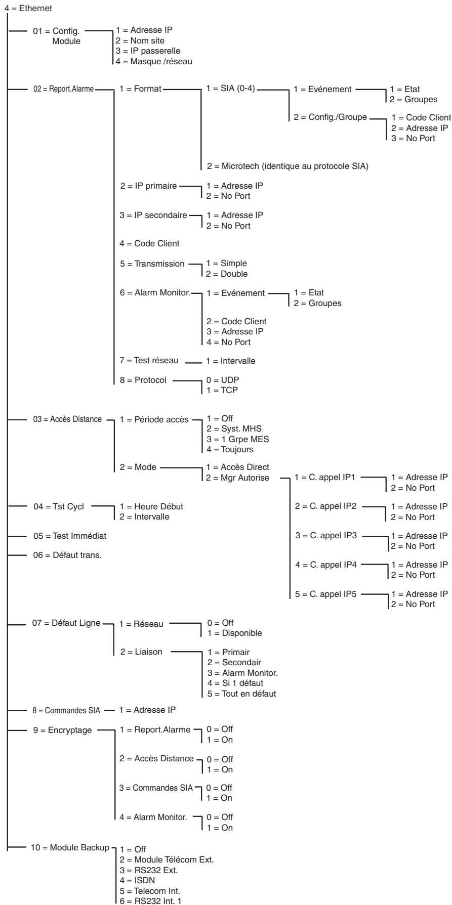
Figure 6-9. Structure de programmation du module Ethernet
