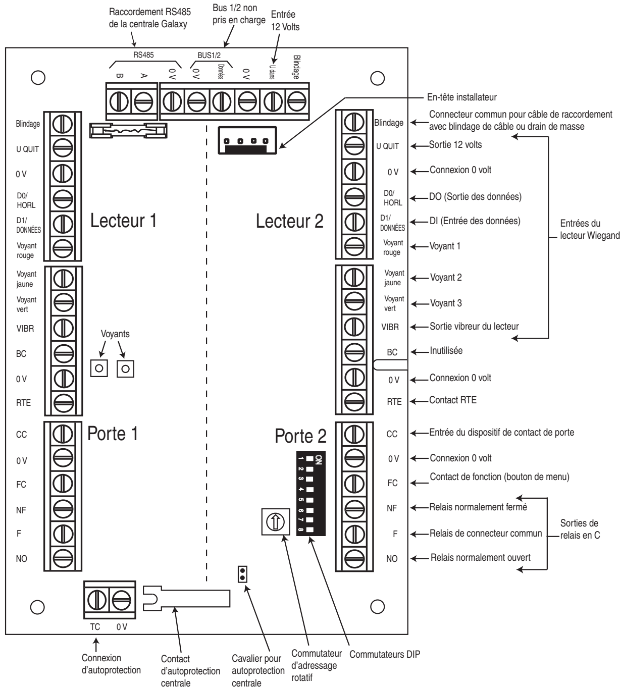
Figure 5-1. Carte électronique du module de contrôle de porte
