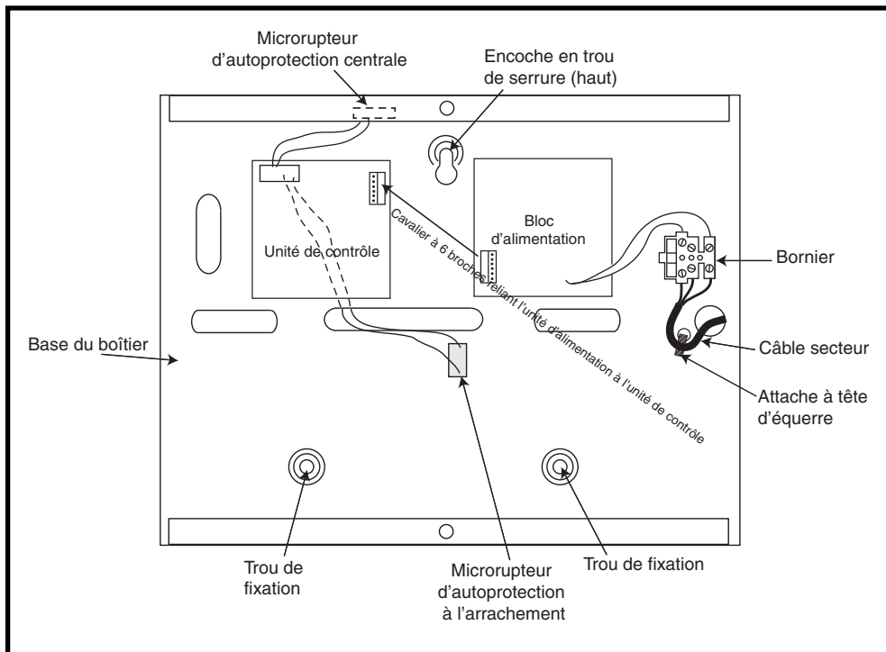
Figure 3-3. Base du boîtier
