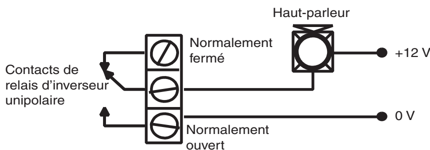
Figure 2-16. Configuration et application standard de sortie de relais d'inverseur unipolaire
