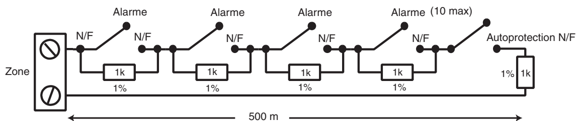
Figure 2-13. Câblage d'une zone vers plusieurs détecteurs
