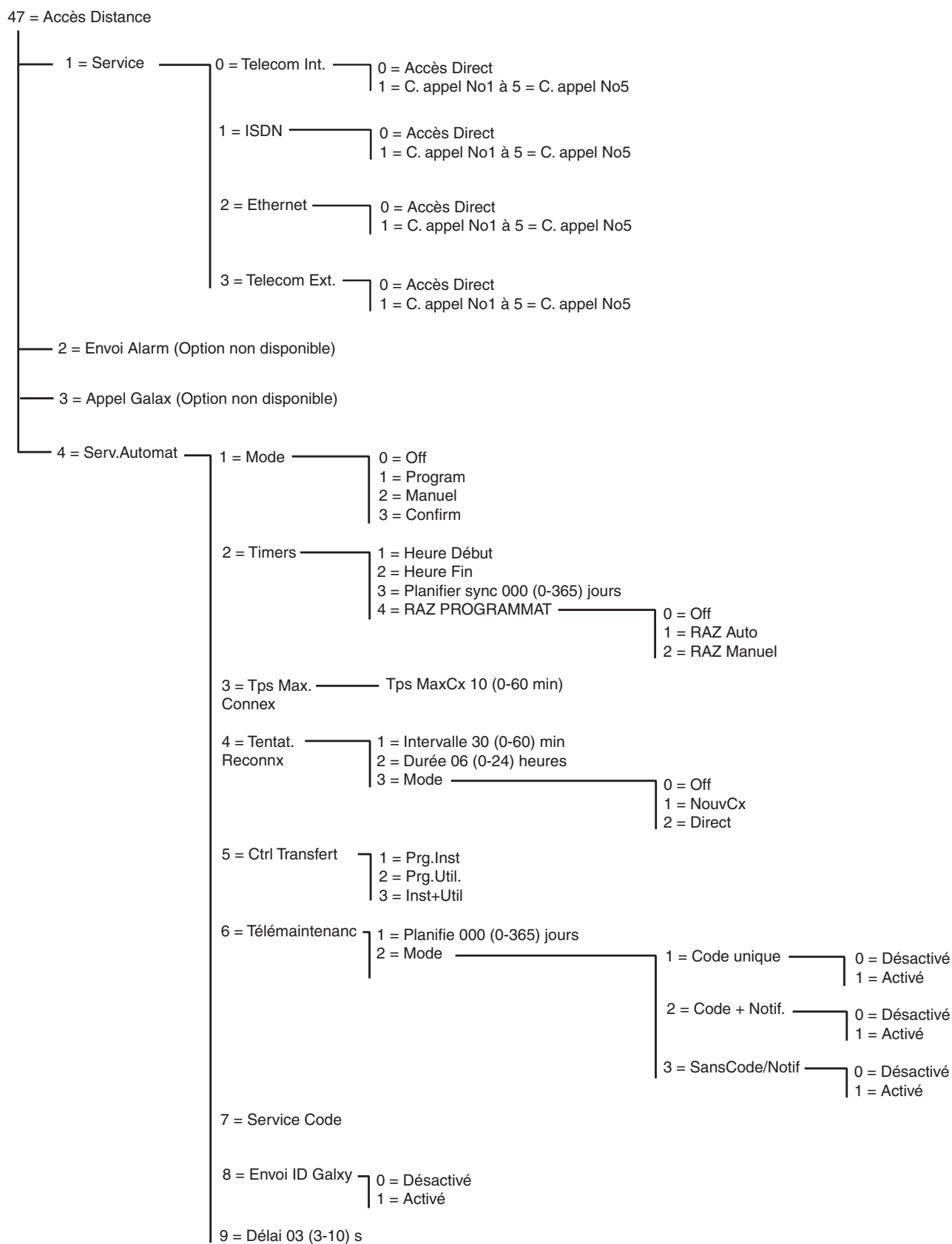
Figure 6-5. Structure d'accès à distance
