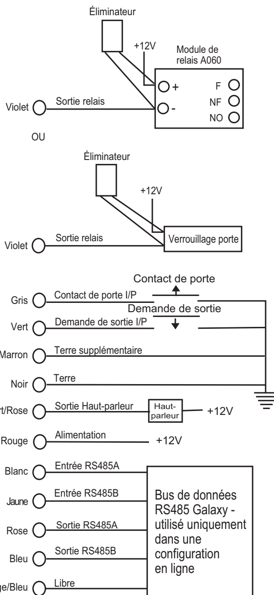
Figure 5-2. Schéma électrique
