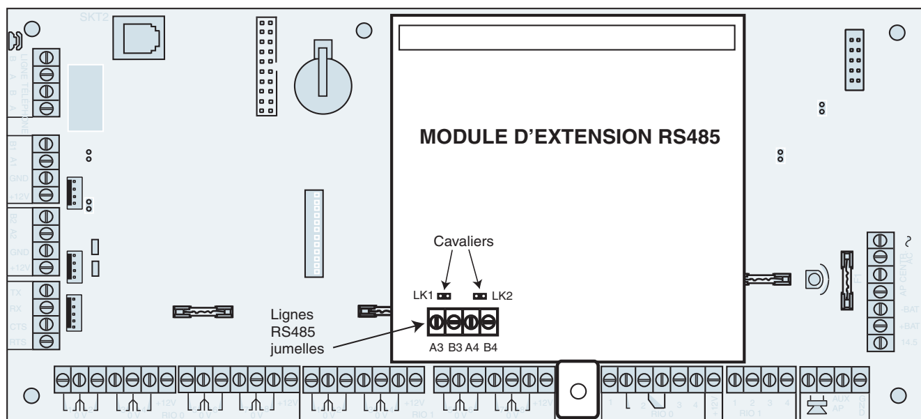
Figure 2-3. Module d'extension RS485
