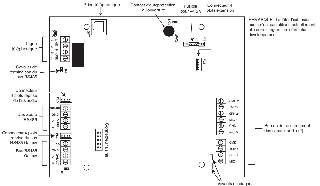
Figure 3-6. Carte électronique de l'interface
