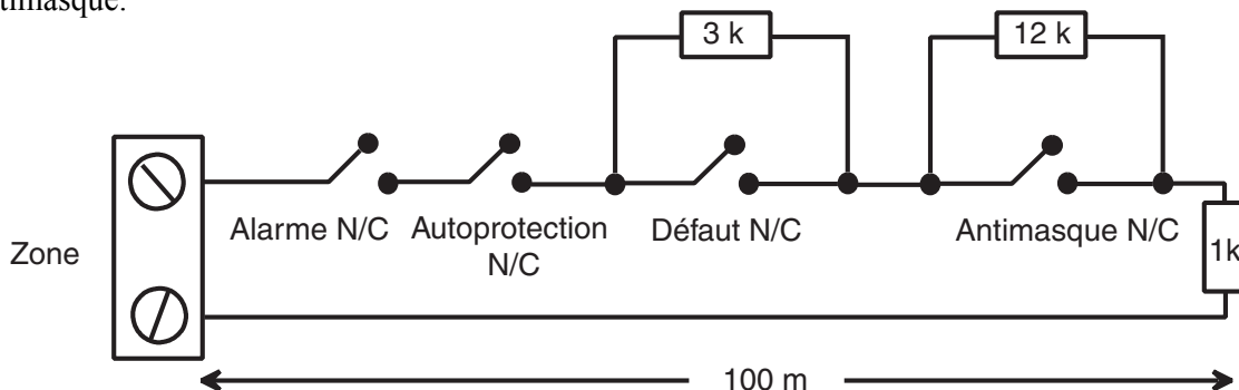
Figure 2-12. Option 10 - Câblage zone/détecteur de fin de ligne
