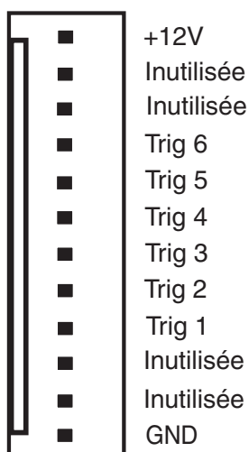
Figure 2-17. Connecteur STU
