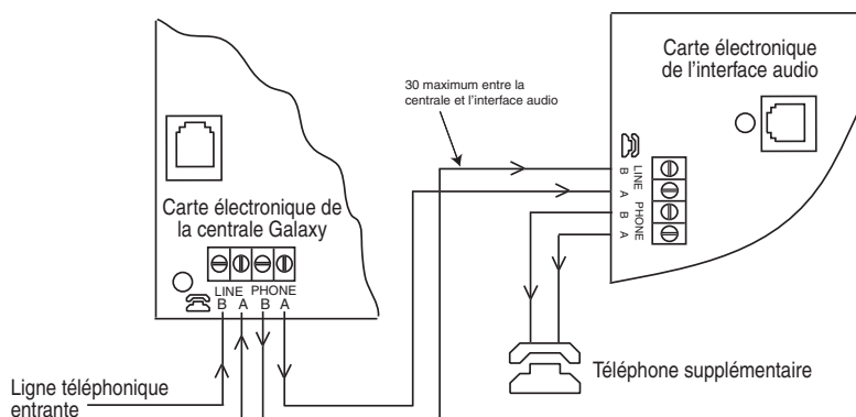
Figure 3-7. Interface audio connecté à la ligne RTC
