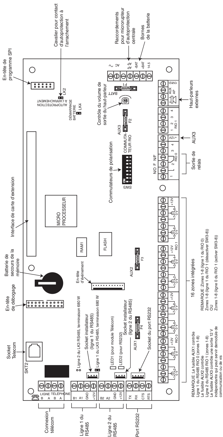
Figure 2-2. Présentation de la carte électronique
