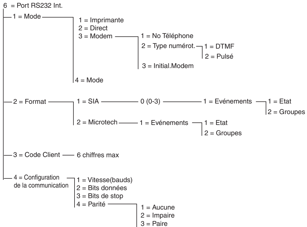
Figure 6-10. Structure de programmation du module RS232 interne
