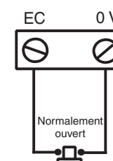
Raccordement du contact de requête de sortie
